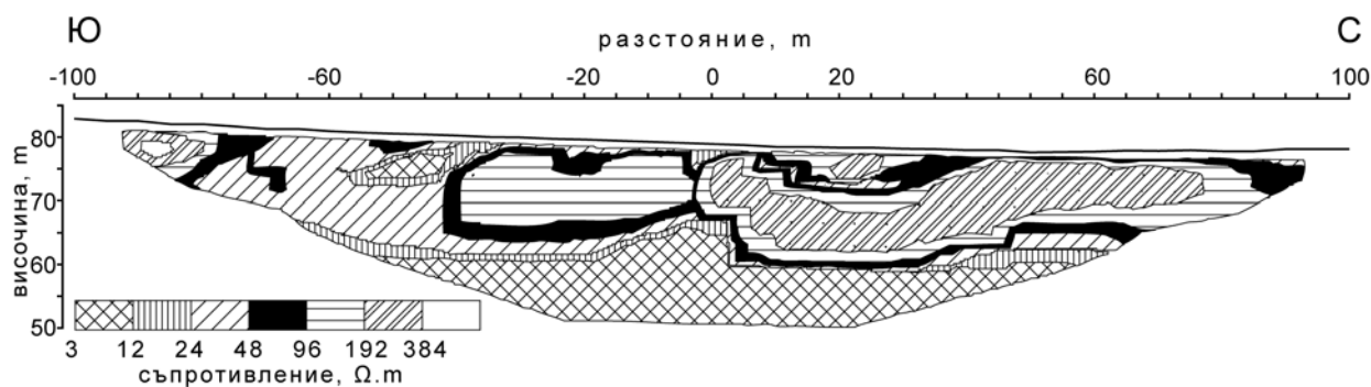
Фиг. 2. Геоелектричен вертикален разрез по профилна линия северно от Харманли. Мястото на профила е посочено със стрелка на фиг.1. Разстояние между електродите 5 м.
